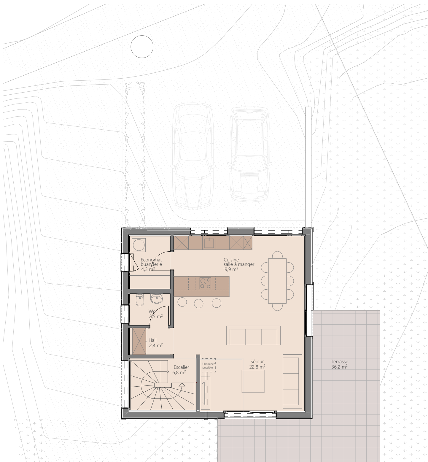
Rez-de-chaussée
